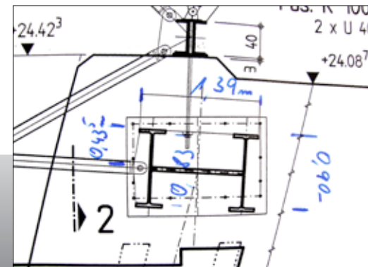
Bauskizze
